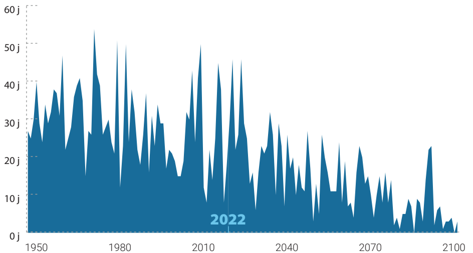
Nombre de jours de gel par an (Tmin < 0 °C) près d'Angers (49)
