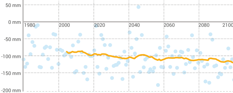
Bilan hydrique (pluie-ETP) pendant le remplissage des grains (variété semis-précoce, semée au 15 avril)
