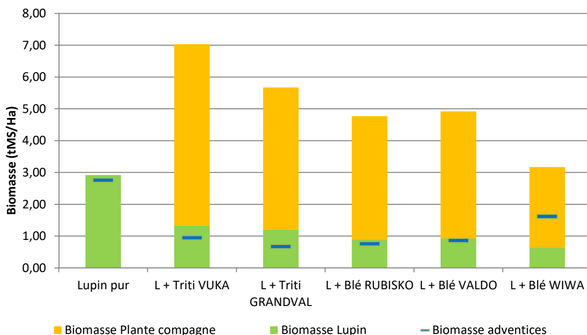
Lupin d'hiver cultivé avec une plante compagne - Vihiers (49) - 2016 Biomasses aériennes à floraison
