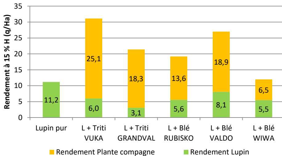
Lupin d'hiver cultivé avec une plante compagne - Vihiers (49) – 2016 Rendements à 15% d'humidité
